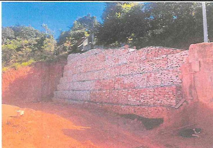
EXECUÇÃO DE GABIÃO-RUA ELZA TEREZINHA- RECANTO DAS ANDORINHAS
