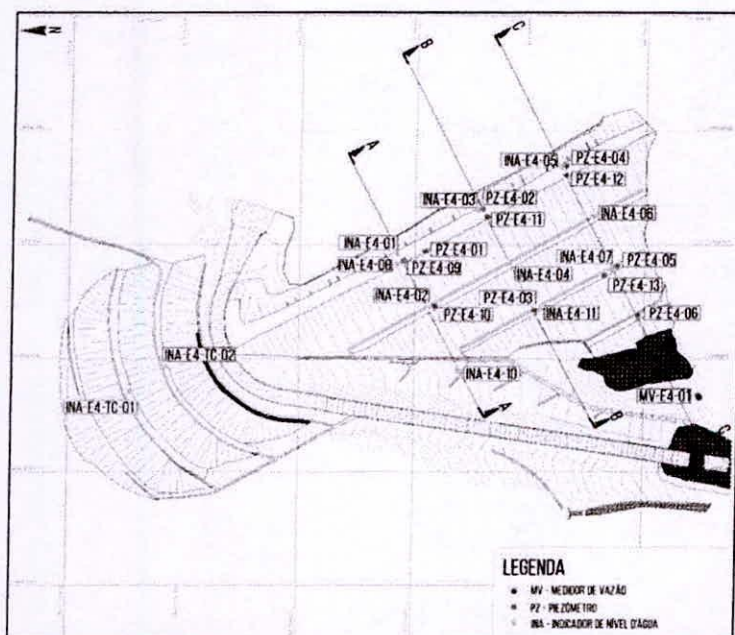
Figura 59 – Planta com a locação da instrumentação existente no dique segundo relatório do checklist .
