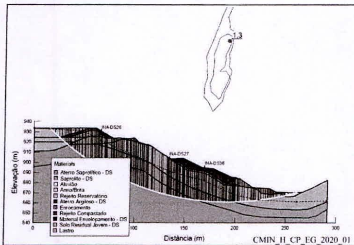
Figura 45 – Seção de estabilidade NN, dique de sela, com detalhe para a cunha de ruptura global passando pelo material Saprólito-Ds.
