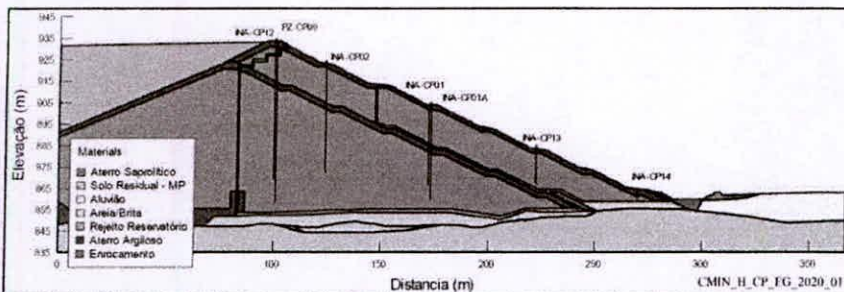
Figura 26 – Seção instrumentada de maior altura do barramento principal (seção CC), com detalhe para a ausência de piezômetros na fundação.
