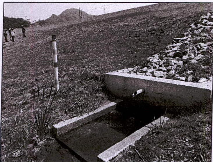
Foto 36 – Saída 02 do dreno de fundo da barragem.
