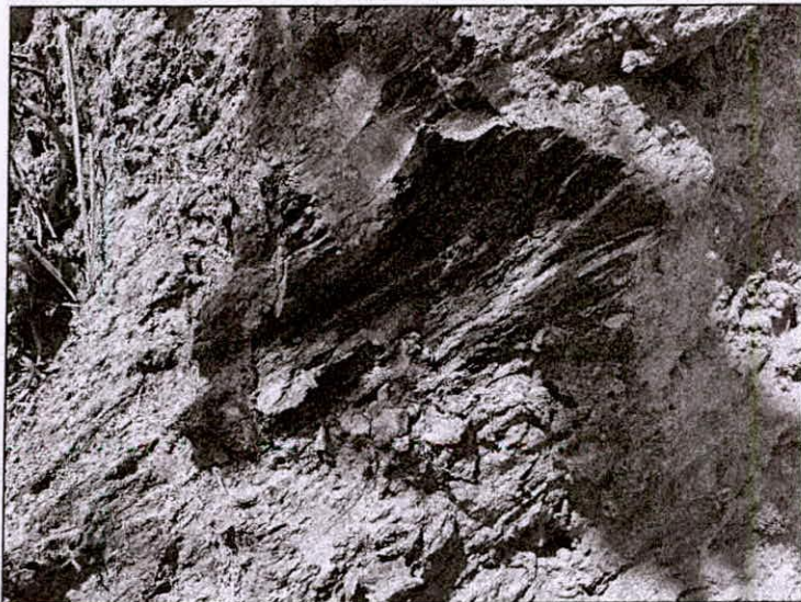
Foto 61 – Detalhe para o material de fundação observado na ombreira esquerda, onde pode se observar que a foliação mergulha em direção favorável à estabilidade da estrutura.
