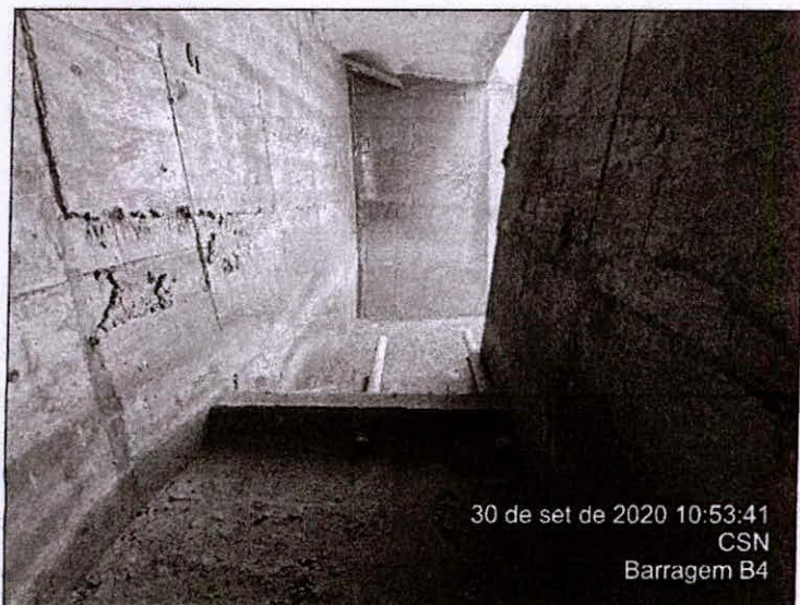
Foto 40 – Vista do desemboque da galeria sob o maciço da barragem.
