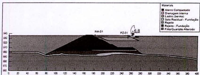
Figura 54 – Seção A-A – Freática definida pelos instrumentos instalados.
