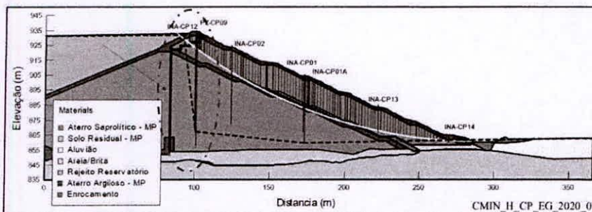
Figura 27 – Seção instrumentada de maior altura do barramento principal (seção CC), com detalhe para a ausência de piezômetros na fundação.
