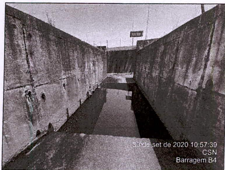
Foto 43 – Bacia de dissipação do sistema extravasador.
