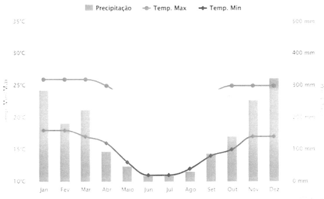
Figura 13 – Histórico climatológico de Congonhas Fonte: ClimaTempo
