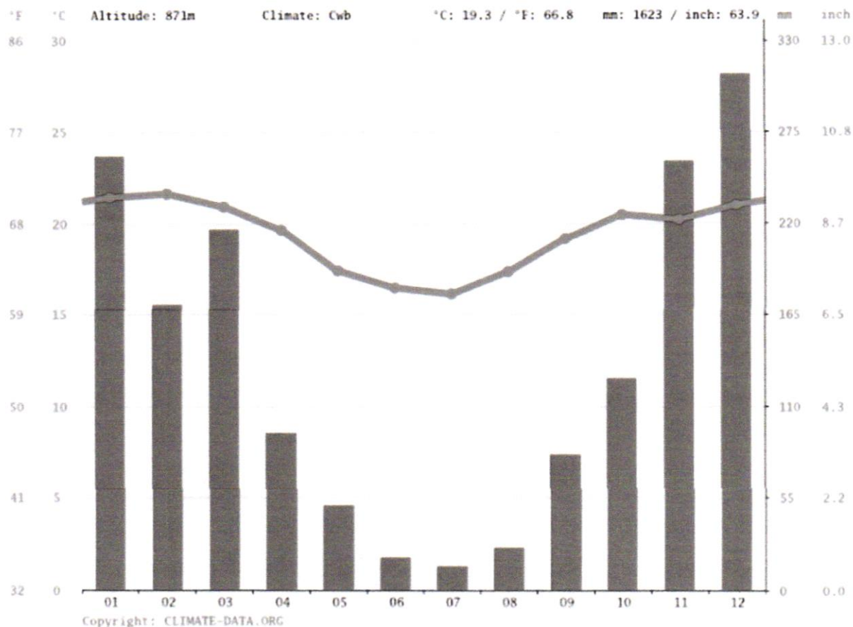
Figura 5: Gráfico anual de precipitação/temperatura do município de Congonhas/MG.
