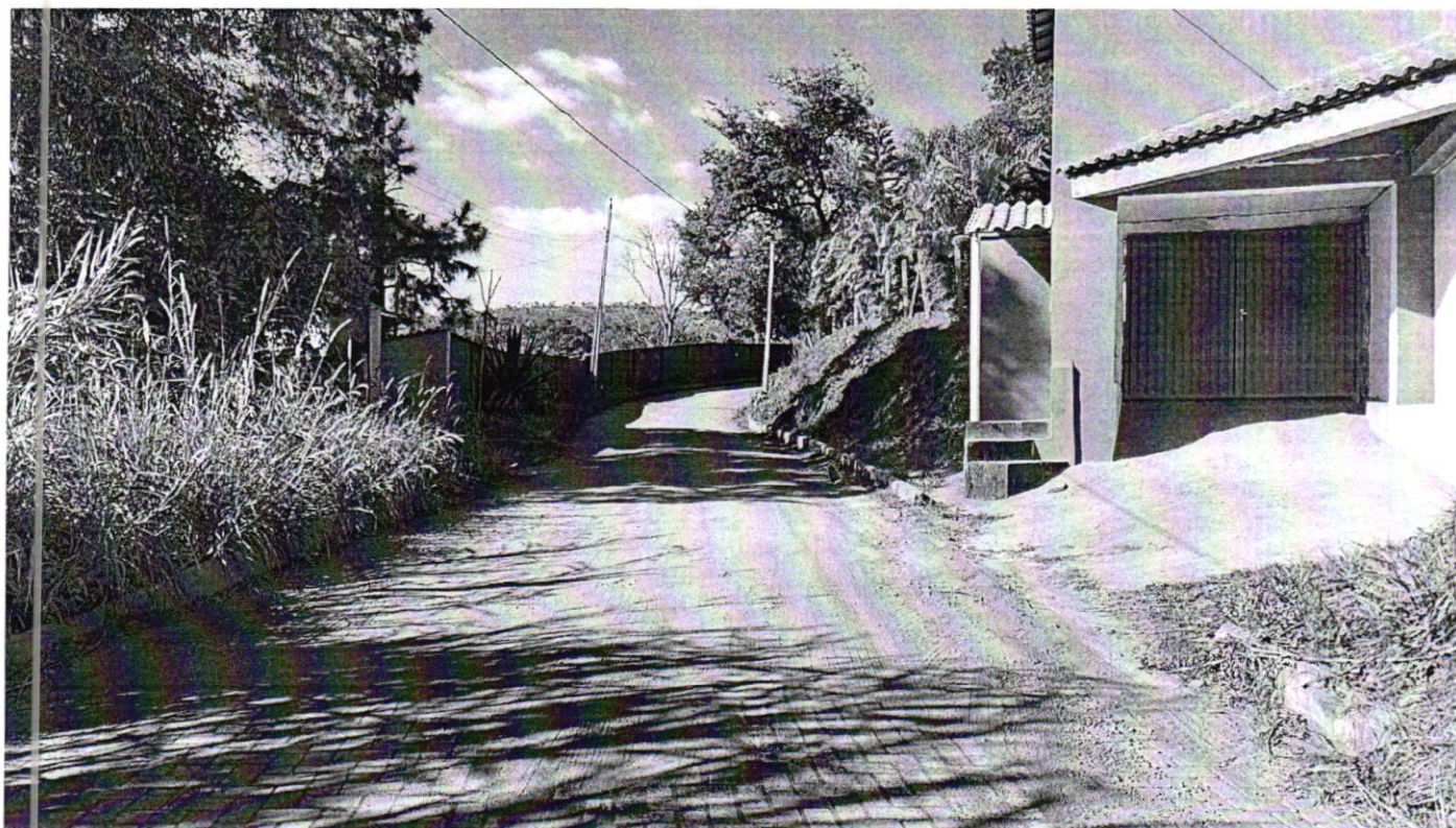
4. Conclusão da pavimentação em blocos intertravados
